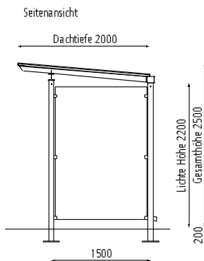
PEGASUS, 2 Felder, mit Dacheindeckung Stahlblechkassetten
