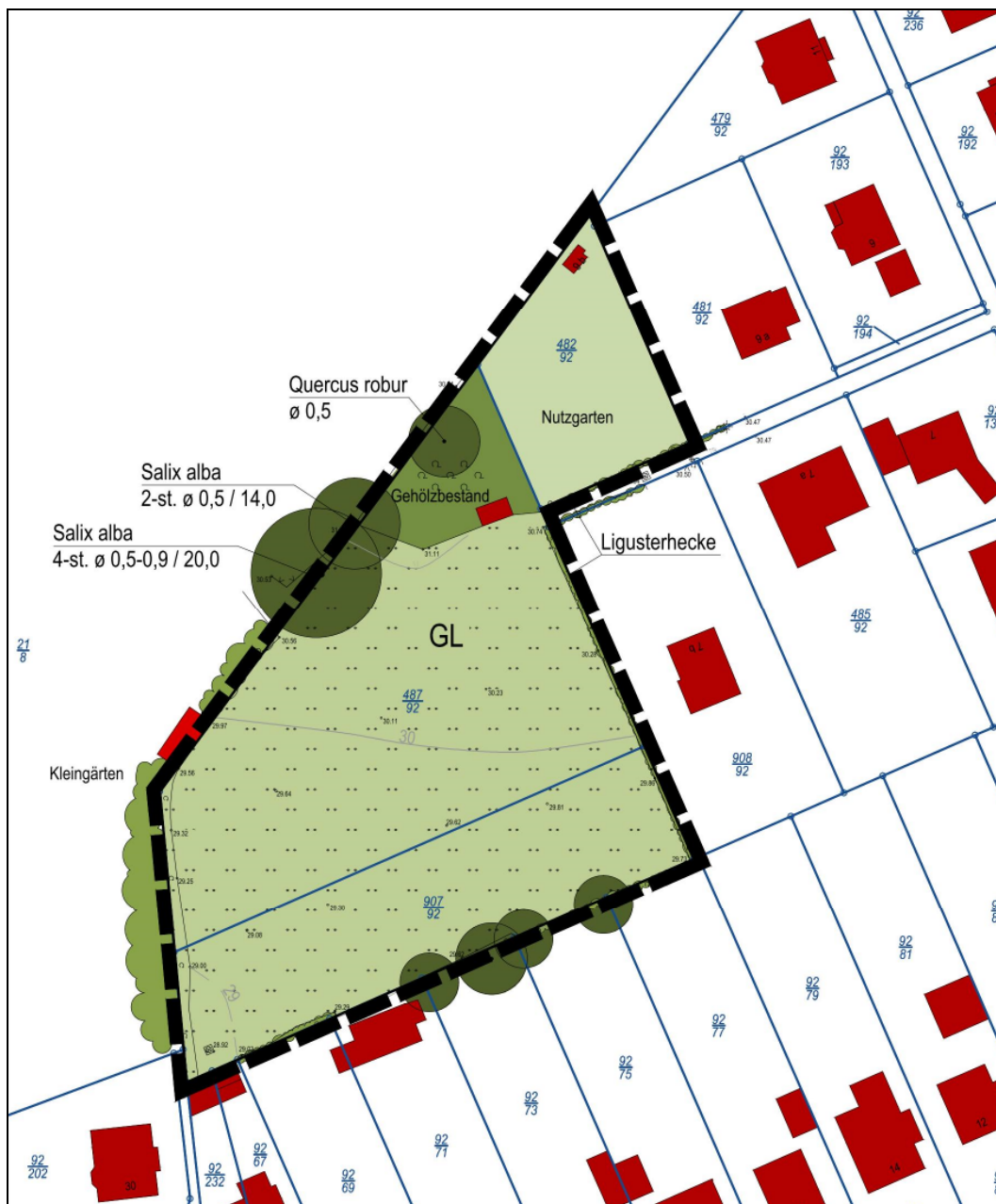
Abb. 8: Bestandsplan o.M.
