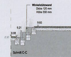
Schnitt C-C'
