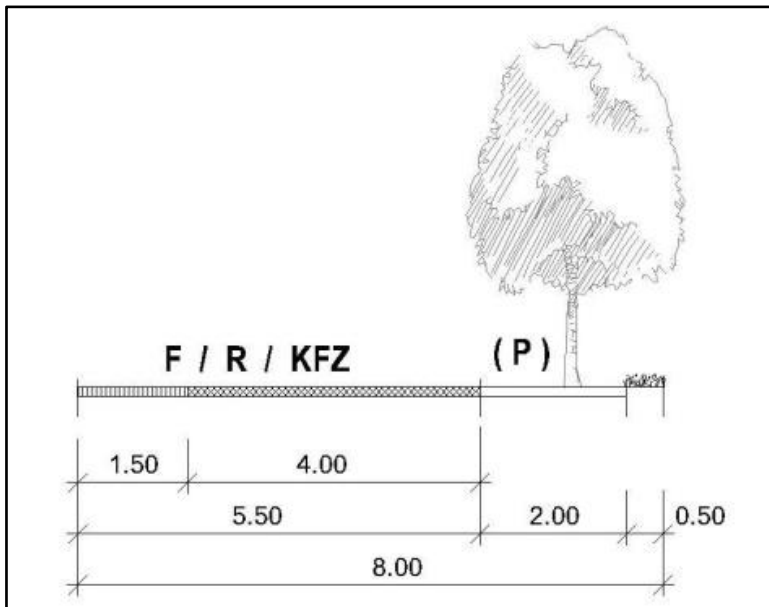
Innere Haupteerschließungsstraße
